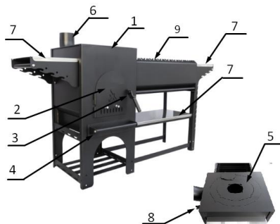
Рисунок 1 Конструктивные элементы печи.
